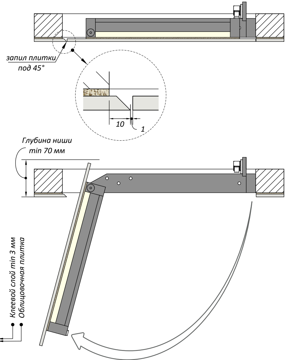
Проем 610 Люк 333 50 10 Ширина плитки 600 мм Высота плитки 300 мм 40 min 1 мм min 1 мм
